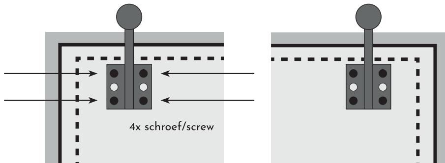
Detail onderaanzicht Bottom view detail
