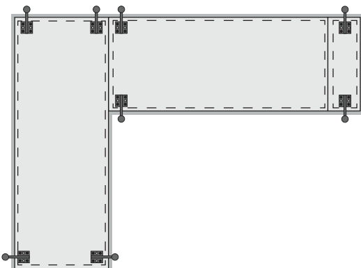
Unterseite Ecksofa Bottom corner sofa
