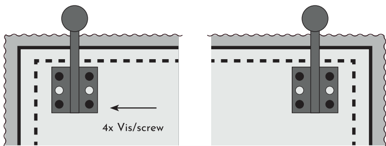
Détail, vu de dessous Bottom view detail
