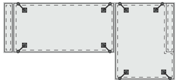
Unterseite Lounge Sofa Bottom lounge sofa
