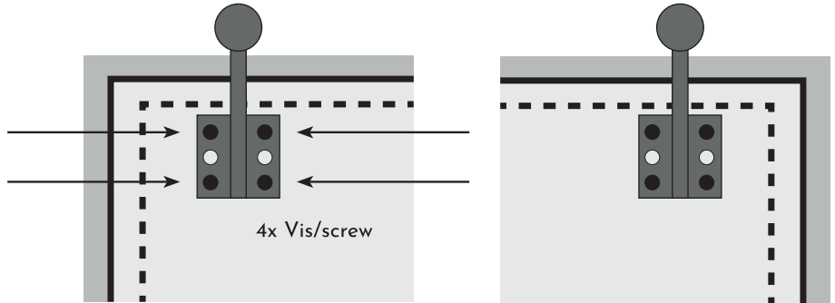
Détail, vu de dessous Bottom view detail
